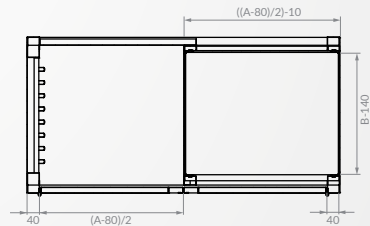
Wymiar półki
