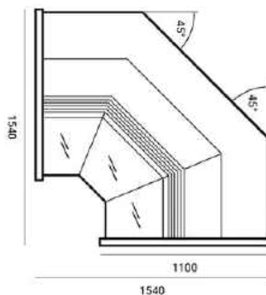
*jedna komora przechowalnicza/one storage chamber
